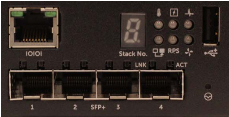
Slika1-2. Dell Networking N1524 Detaljan prikaz
