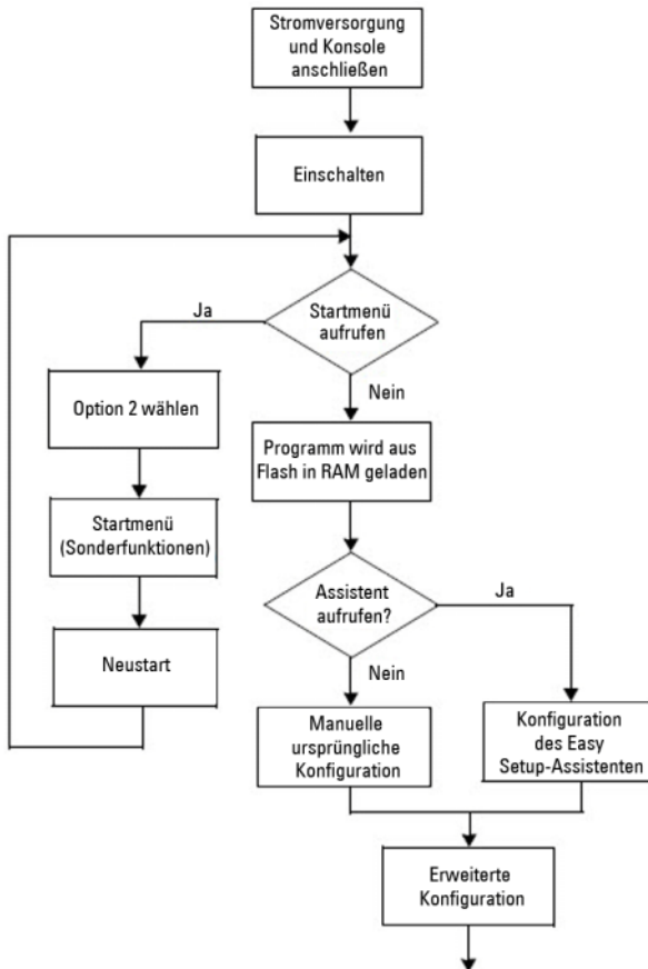
Abbildung 1-8. Flussdiagramm für Installation und Konfiguration
