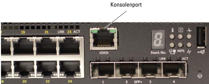
Abbildung 1-9. N1524P Frontblende mit Konsolen-Port
