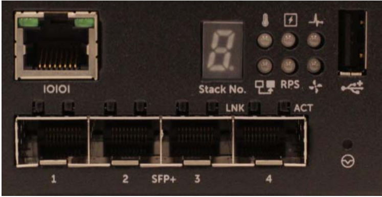
Şekil 1-2. Dell Networking N1524Yakından bakış
