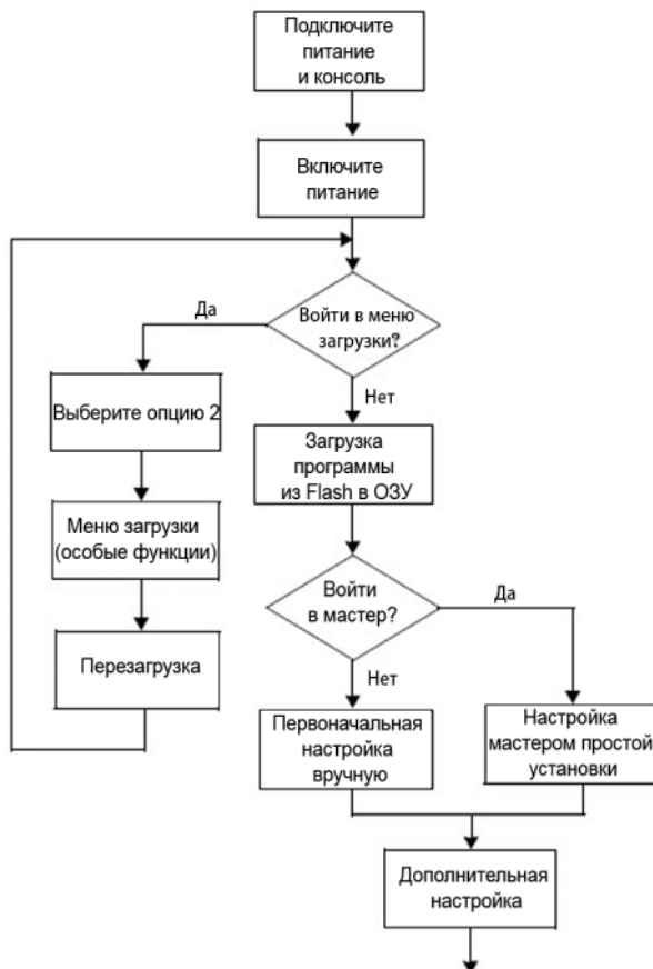
Рисунок 1-8. Установка и настройка блок-схемы
