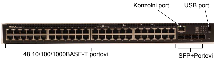
Slika1-1. Dell Networking N1548 sa 48 10/100/1000BASE-T portovima (prednja ploča)
