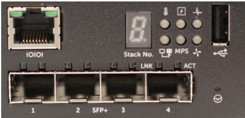
Slika1-3. Dell Networking N1524P Detaljan prikaz
