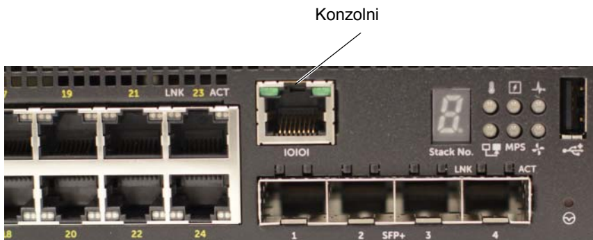
Slika1-9. N1524P Prednja ploča sa konzolnim portom
