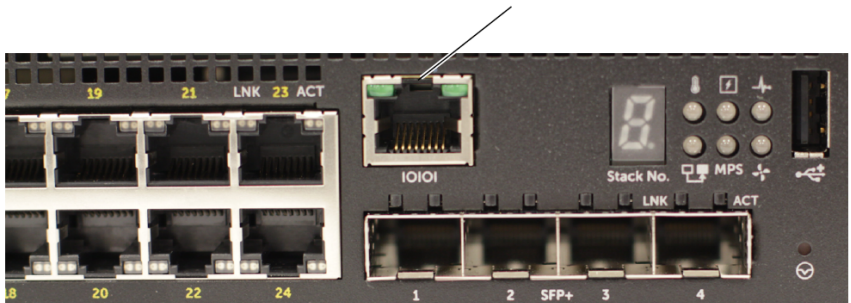
איור 1-9 לוח קדמי של N1524P עם יציאת מסוף בקרה
