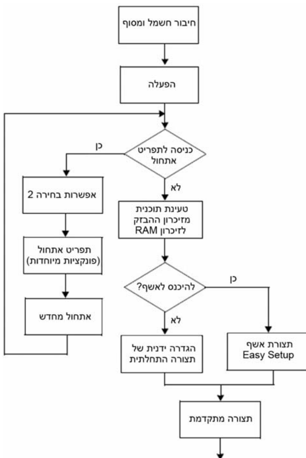
איור 1-8 תרשים זרימה להתקנה וקביעת תצורה
