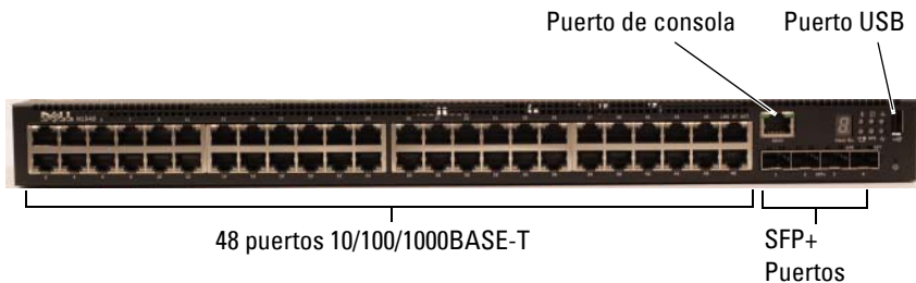
Ilustración 1-1. Dell Networking N1548 con 48 puertos 10/100/1000BASE-T (panel frontal)
