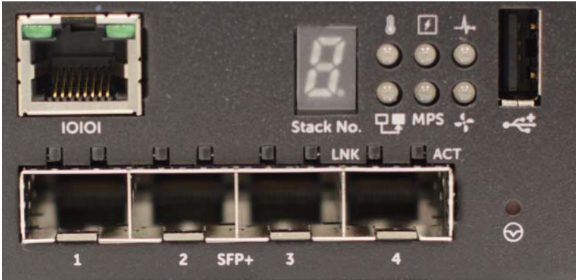
Şekil 1-3. Dell Networking N1524PYakından bakış
