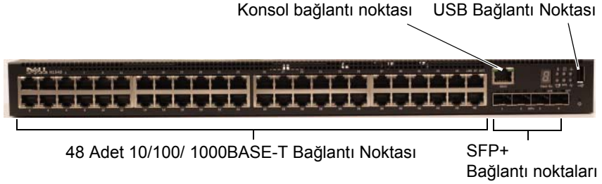
Şekil 1-1. Dell Networking N1548 48 10/100/ 1000BASE-T Bağlantı Noktaları (Ön Panel)
