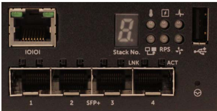
Рисунок 1-2. Dell Networking N1524 (крупным планом)
