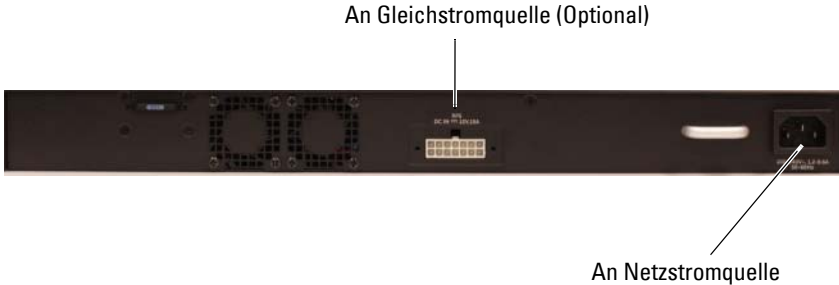
Abbildung 1-10. Wechselstrom- und Gleichstromanschluss ein einen N1548 Switch
