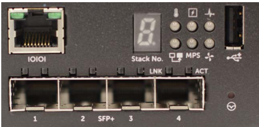
Ilustración 1-3. Primer plano de Dell Networking N1524P
